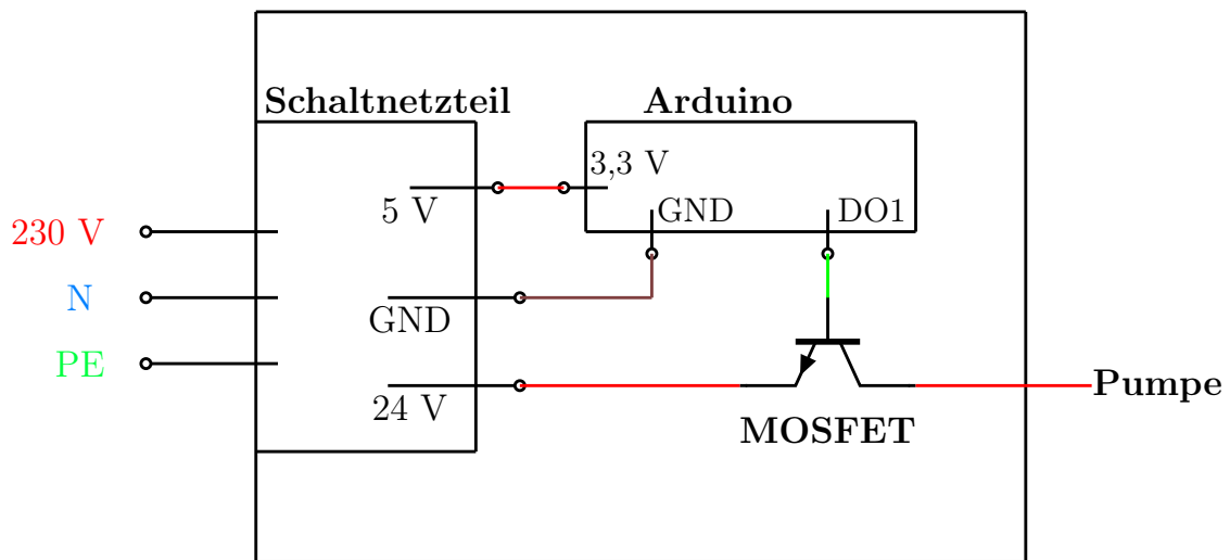
Abbildung 3.2: Der Netzteilkasten
